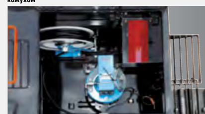
Электрический шприц-пистолет для консистентной смазки с барабаном для шланга (опционно)
