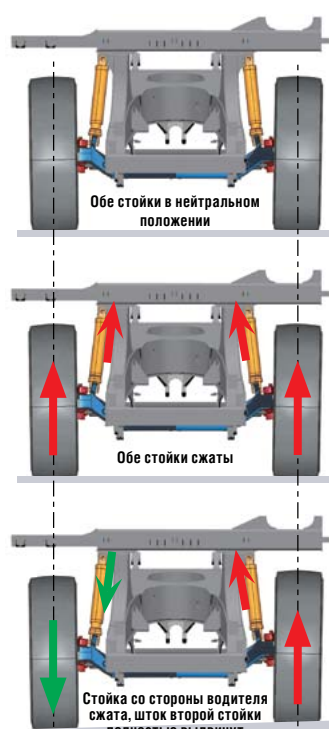
Подвеска на продольных рычагах (передняя)
